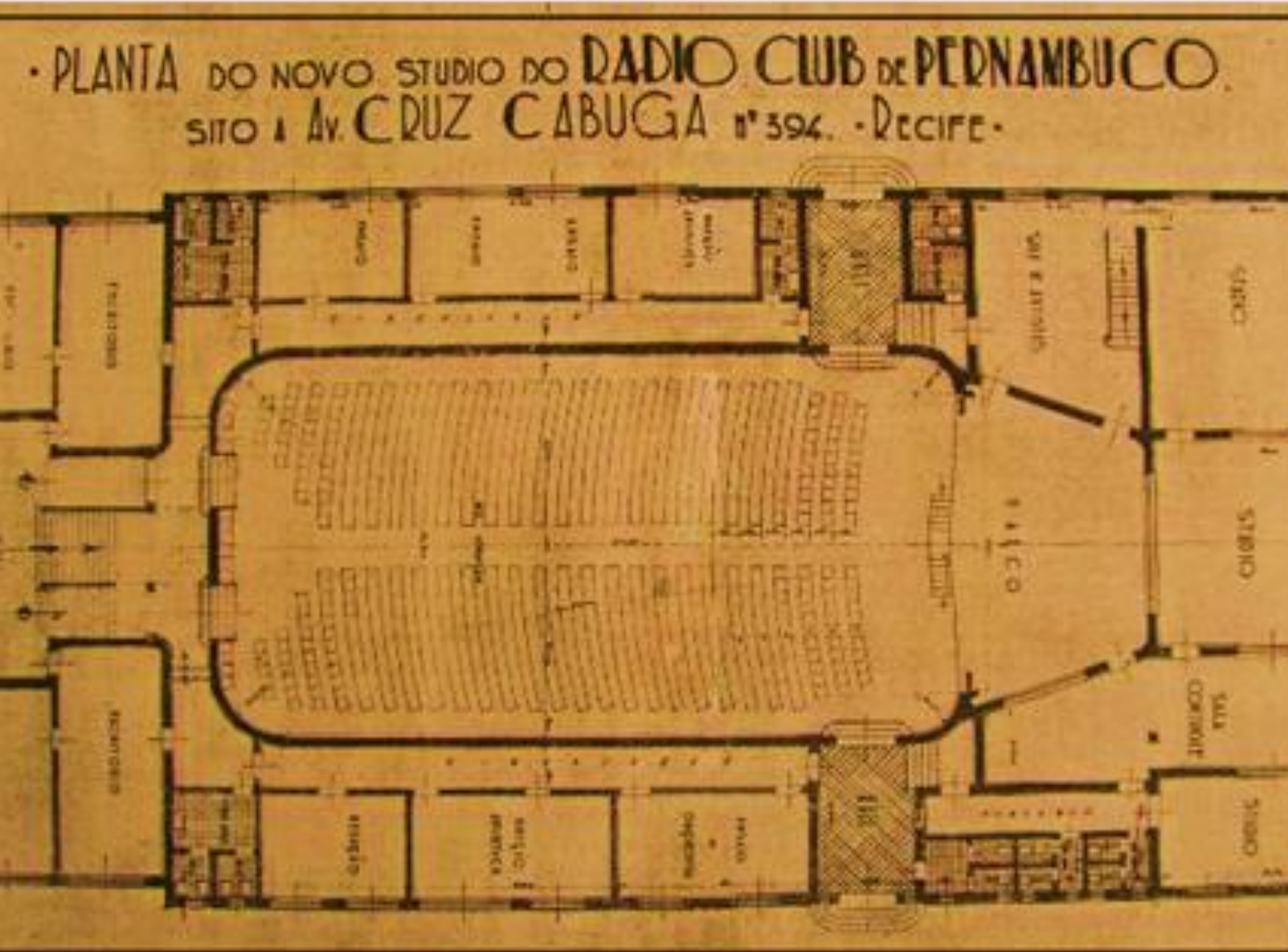
Planta do estúdio da Rádio Clube de PE (1950)
